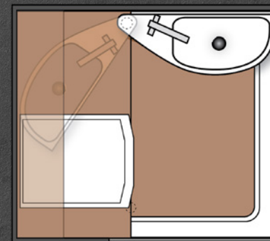
LAYOUT WC a separazione secca
